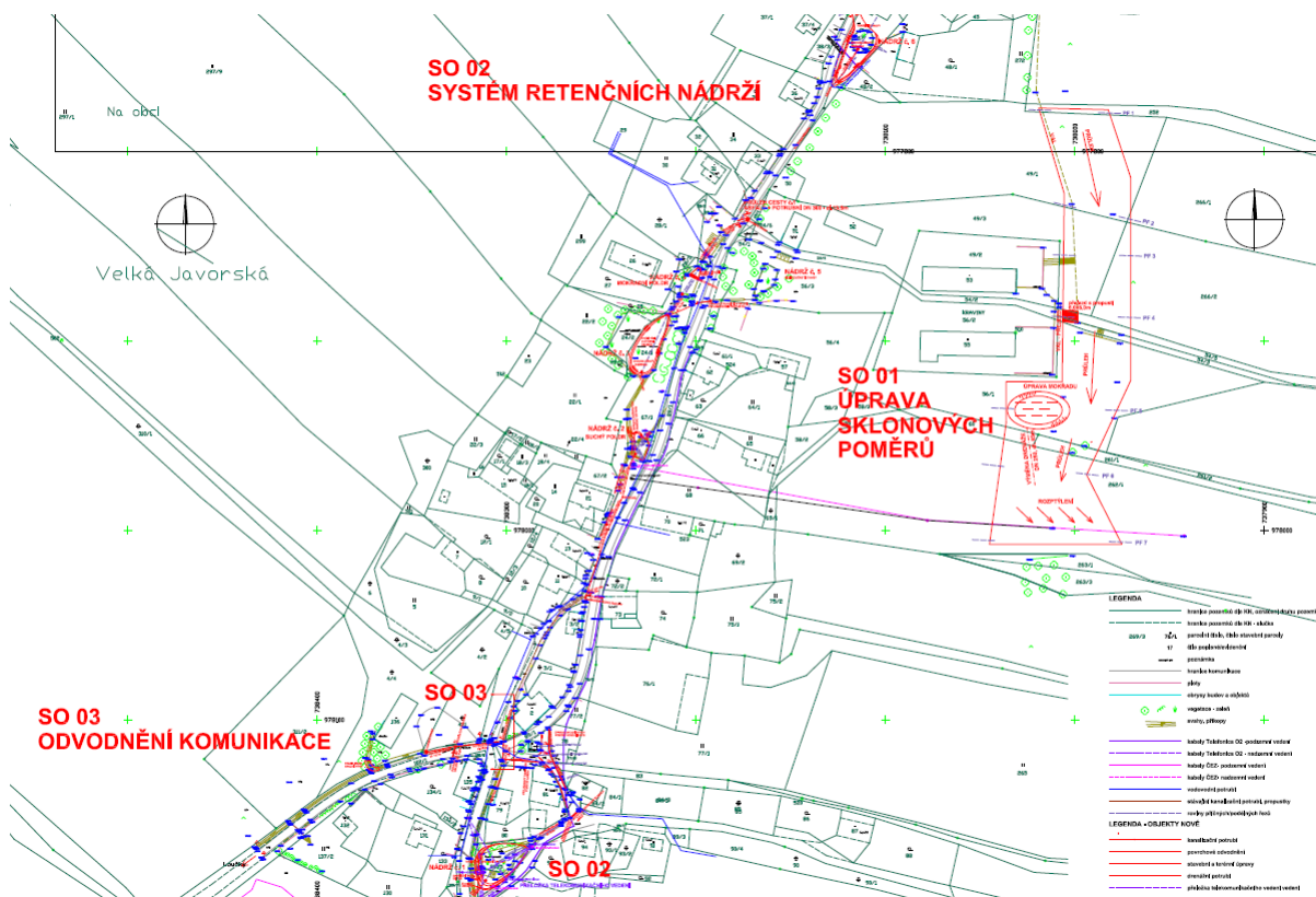
Obr.: Záměr revitalizace soustavy rybníků ve Velké Javorské
